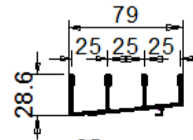
R2 Kisko-4 18163ER
