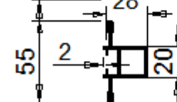
R6A Pysty, 2-laippainen 18168
